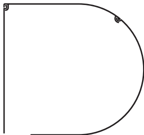
Formado SGF Mögliche Kastengrößen in mm: 125, 137, 150, 165, 180, 205
