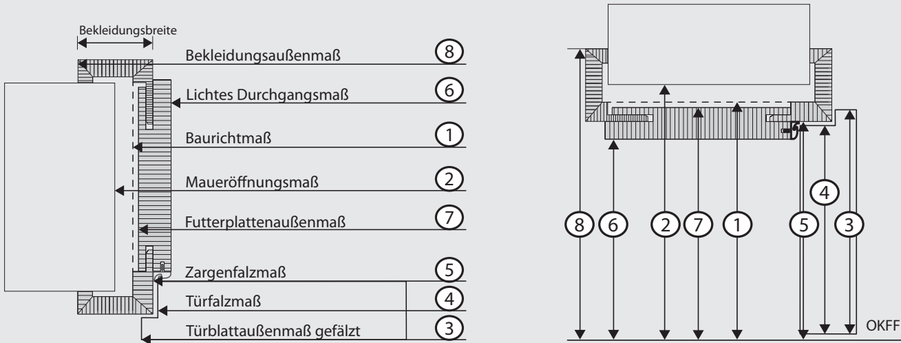
DIE WICHTIGSTEN MAßE AUF EINEN BLICK Darstellung: Gefälztes Türelement
