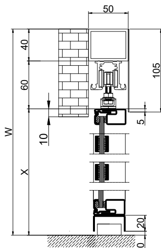
Wandmontage / Sturz
