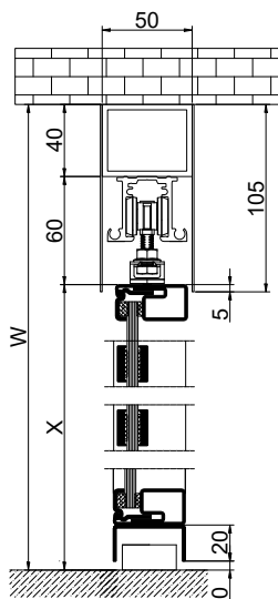
Deckenmontage
